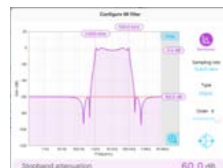
Digitale filterbox
